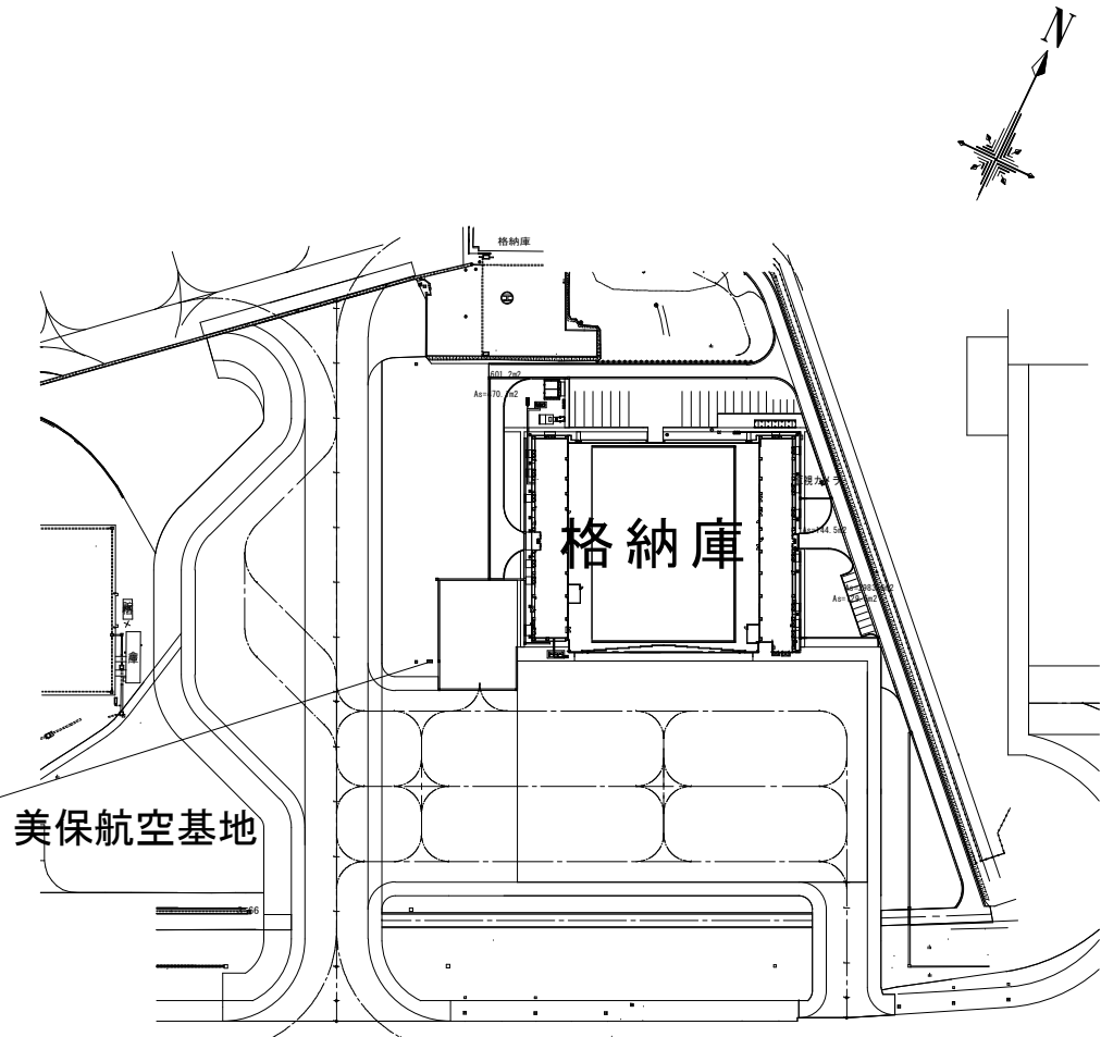
美保分屯地 油分離槽配置図
