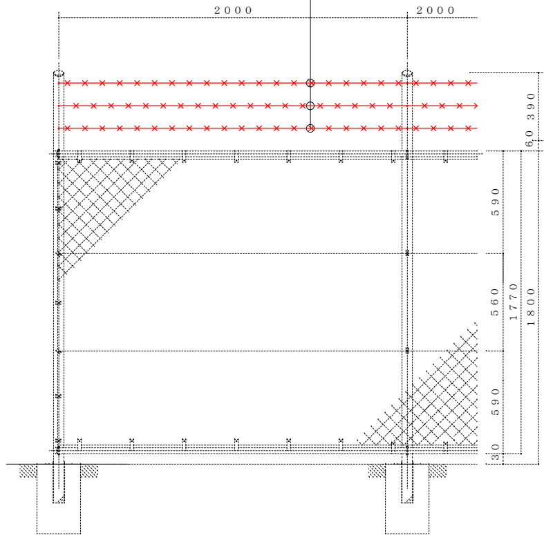
フェンス標準図 S=1/30
