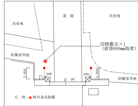
配置図 S=1/500
