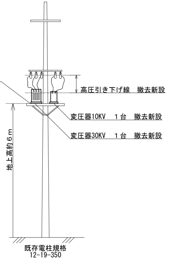
給油所西側 立面図 S=1/100
