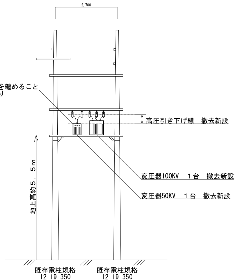
101号庁舎北側 立面図 S=1/100
