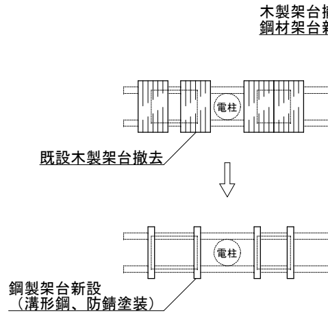
架台平面図 S=1/40
