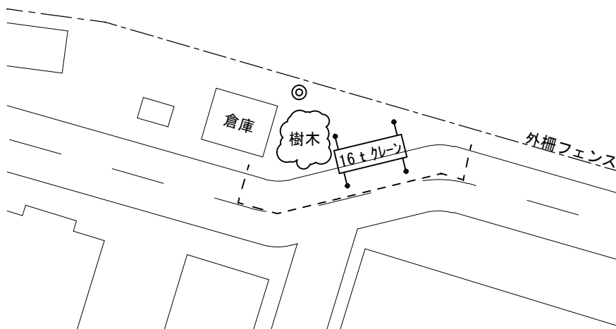
101号庁舎北側 作業場所 平面図 S=1/500
