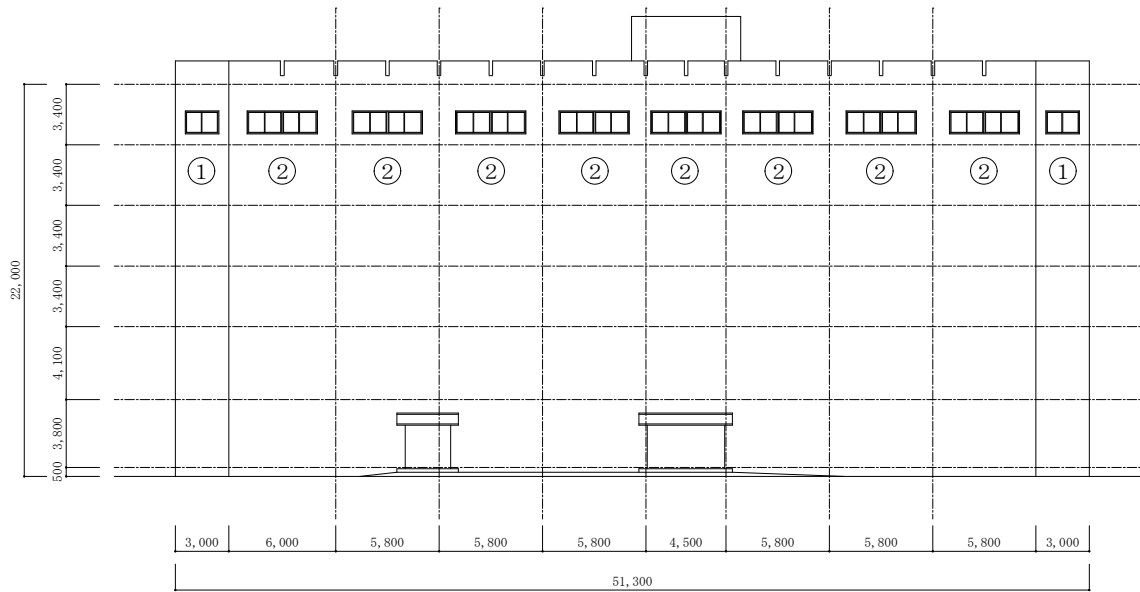
87号隊舎南側立面図
