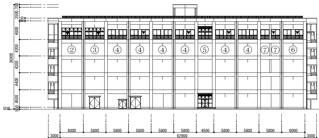
103号隊庁舎北側立面図
