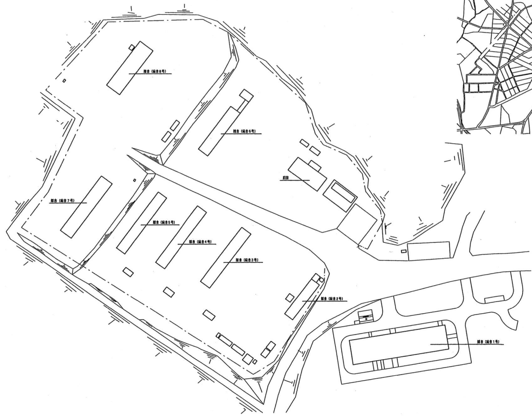
配置図 1/750
