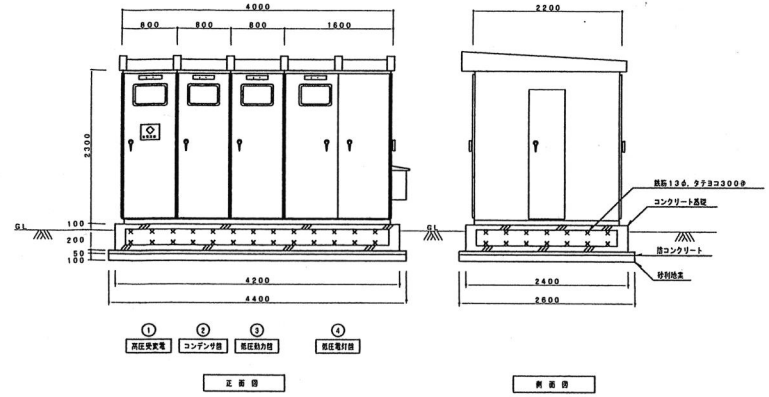
展覧型キュービクル (参考) 姿図 (コンクリート基礎 木工事)
