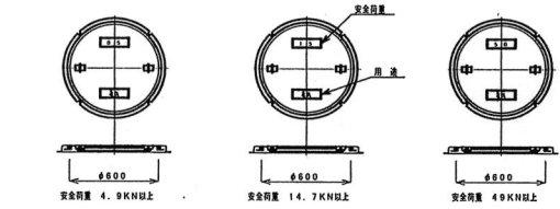
鎖・ゴムパッキング取付図
