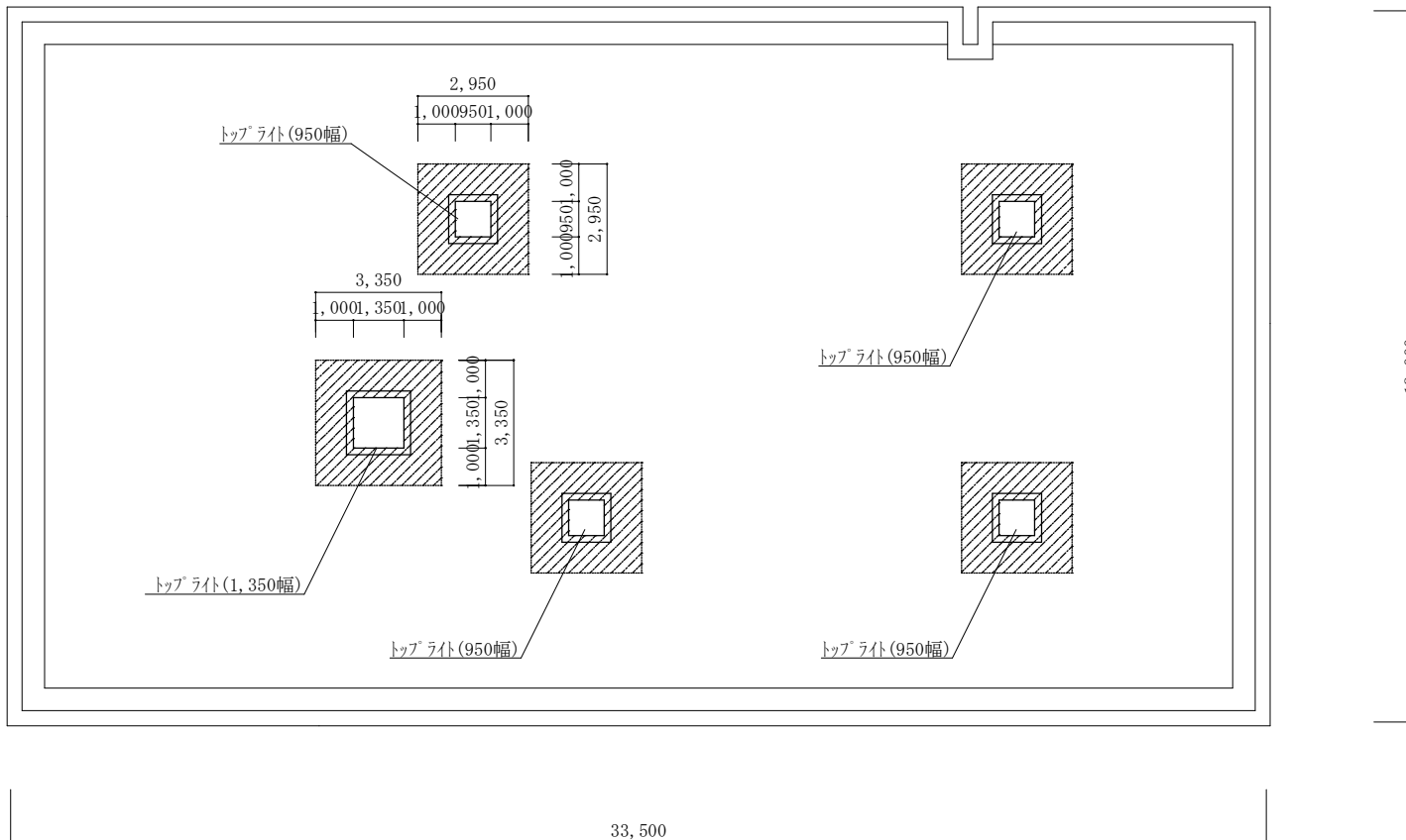
221号建物屋外平面図 S=1:200
