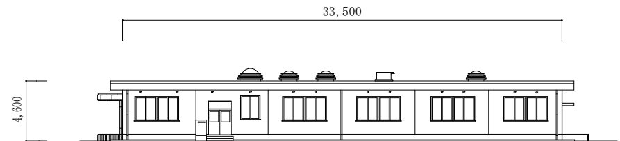
221号建物立面図 S=1 : 400
