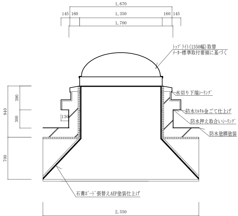
トップライト(1,350幅)詳細立面図 S=1:30
