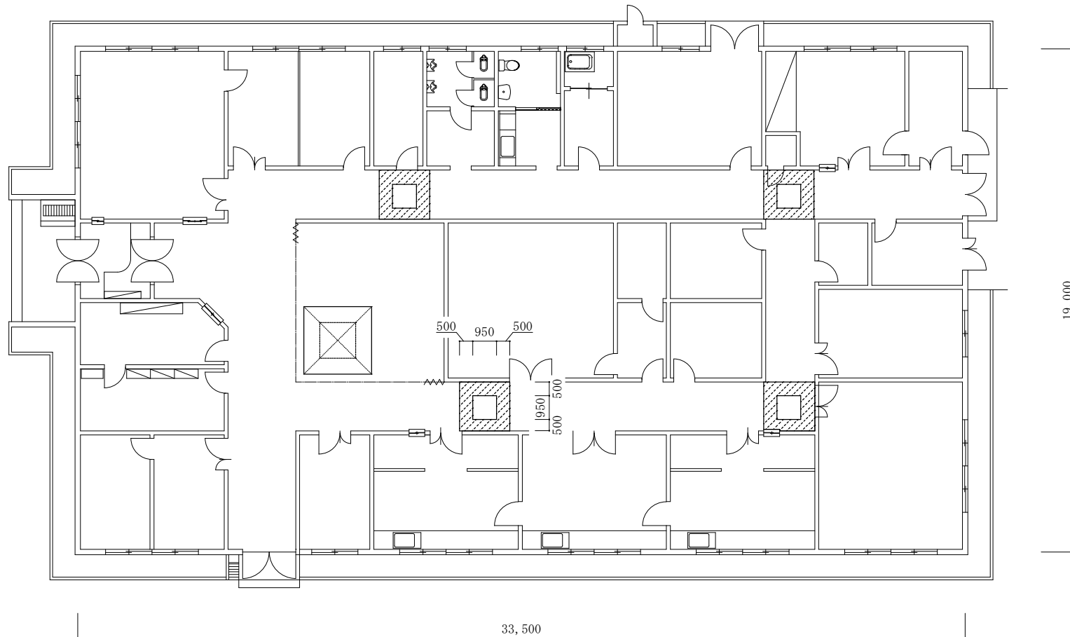
221号建物屋内平面図 S=1:200
