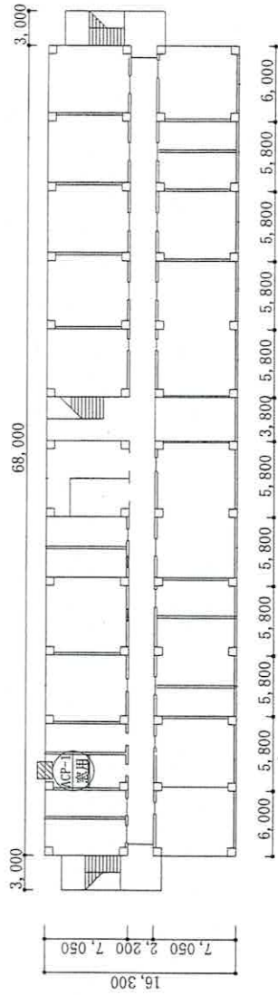
陸上自衛隊山口駐屯地本庁舎3F平面図 1/500
