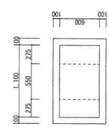
洗車場油分離槽 S=1:50
