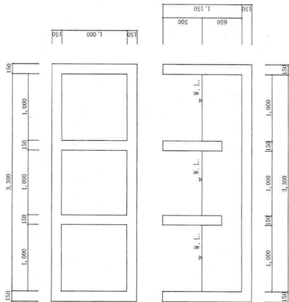
むつみ演習場厨房油分離槽 S=1:50
