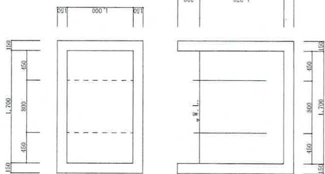
むつみ演習場洗車場油分離槽 S=1:40
