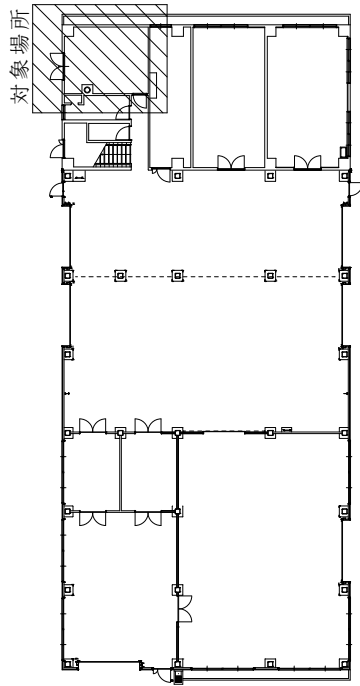
272号建物1階平面図 S=NoScale
