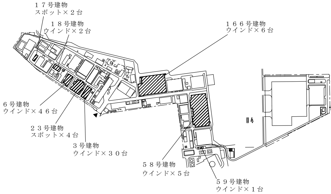
配置図 1 : 7500
