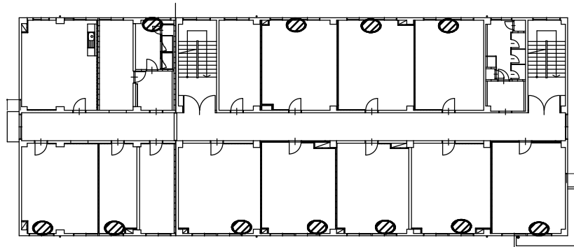
3号建物 2 F 平面図 窓枠 h = 1.8m 計 11 台
