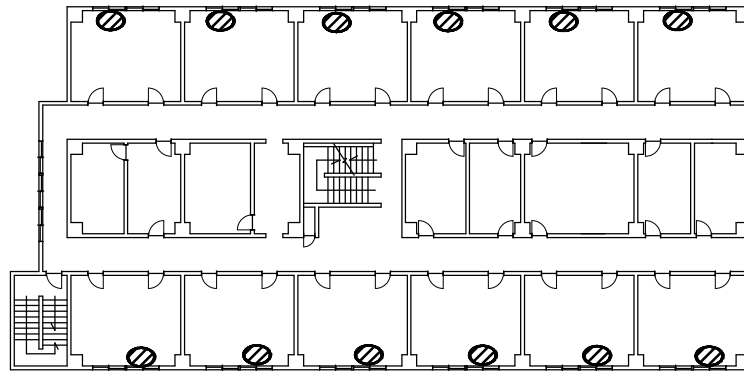
6号建物 4 F 平面図 窓枠 h = 1.3m 計 12 台
