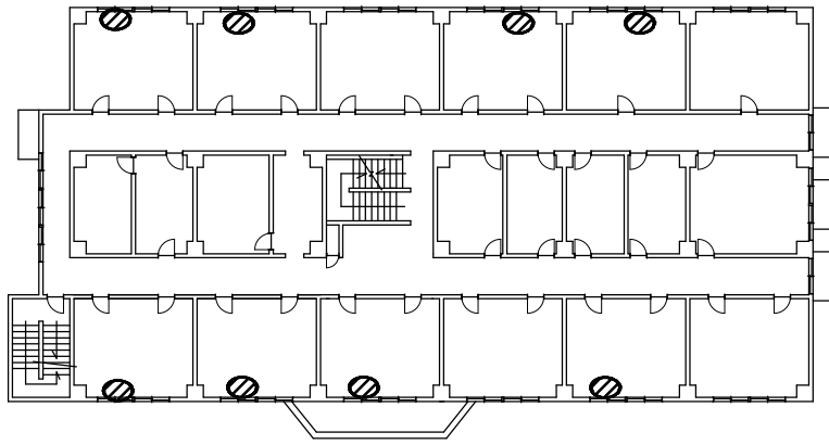
6号建物 2 F 平面図 窓枠 h = 1.3m 計 8 台
