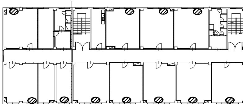
3号建物 3 F 平面図 窓枠 h = 1.8m 計 11 台
