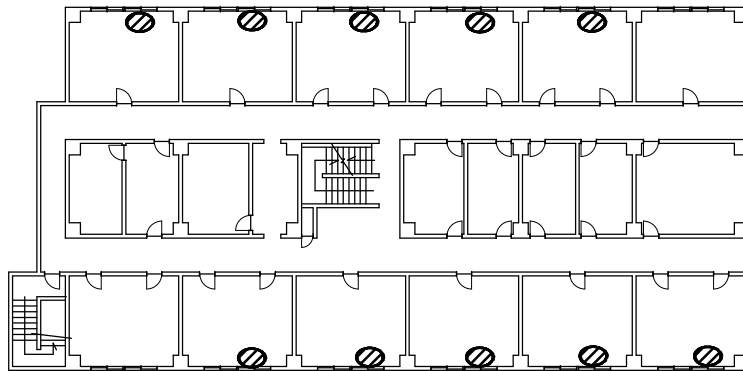
6号建物 5 F 平面図 窓枠 h = 1.3m 計 10 台
