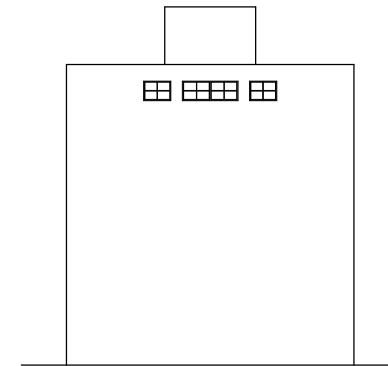
194号隊舎西側立面図
