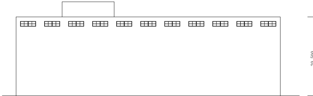
194号隊舎北側立面図
