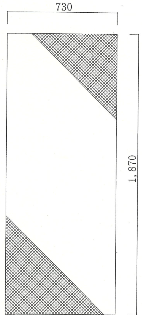
詳細図 S=1/150
