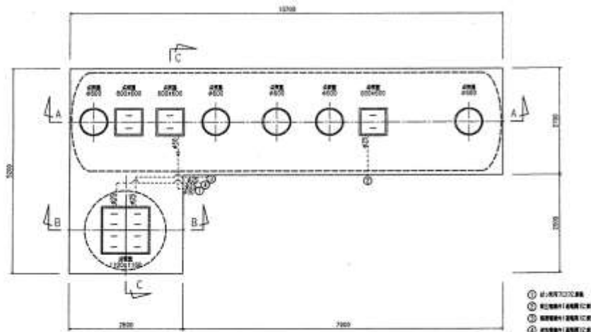
スラブ平面図 1/150
