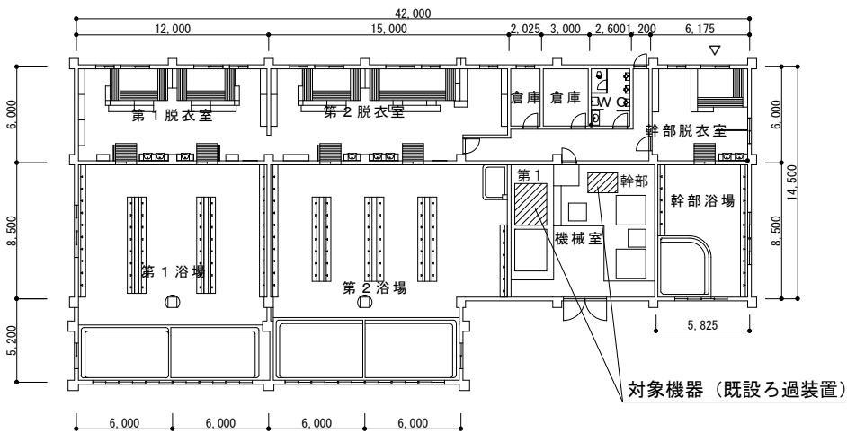
浴場平面図 S=1/300
