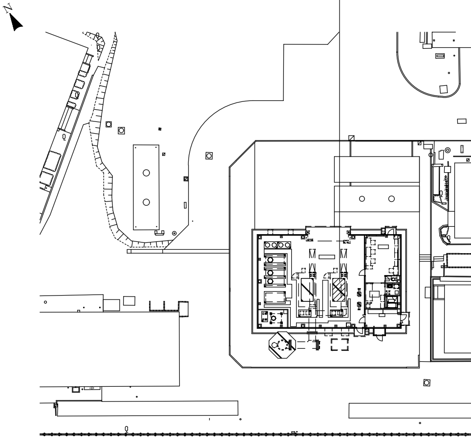
110号ボイラー室平面図 S=1/150
