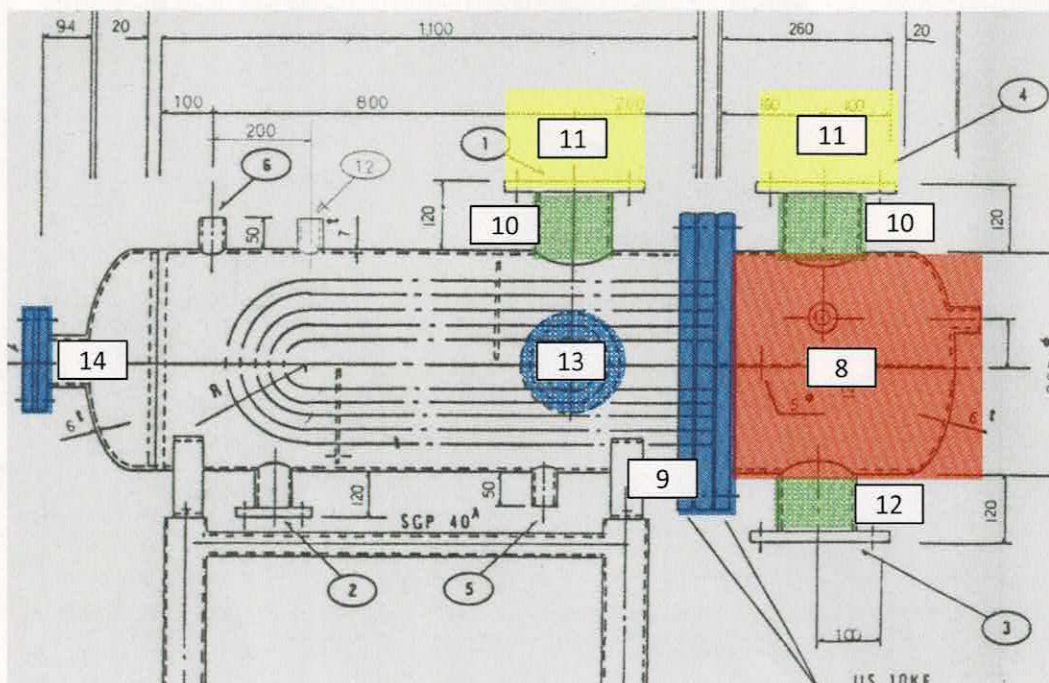
熱交換器
