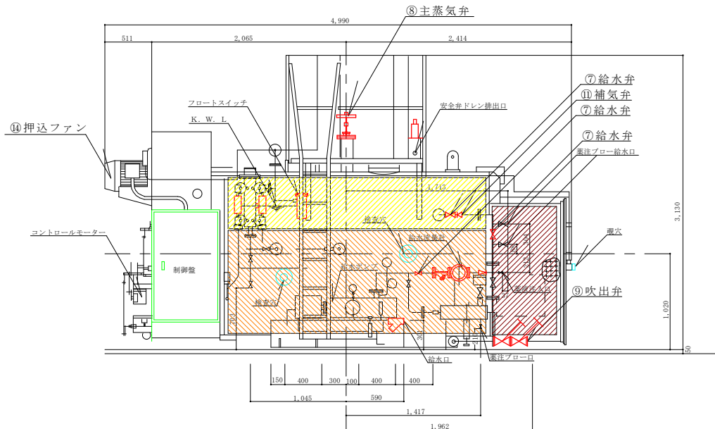
ボイラー本体側面図
