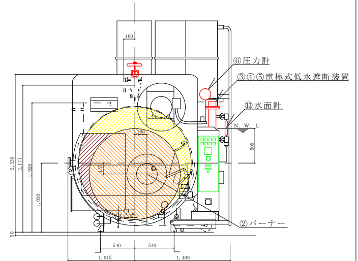
ボイラー本体正面図
