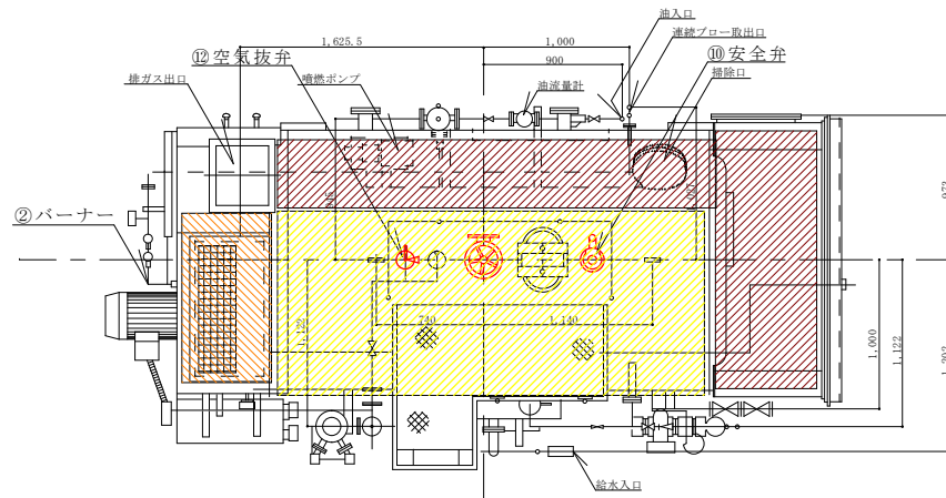
ボイラー本体上面図
