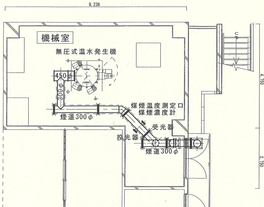
機械室平面詳細図 (1/100)
