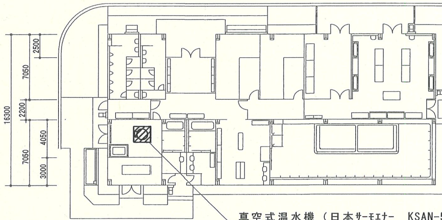
演習場浴場平面図 1/400
