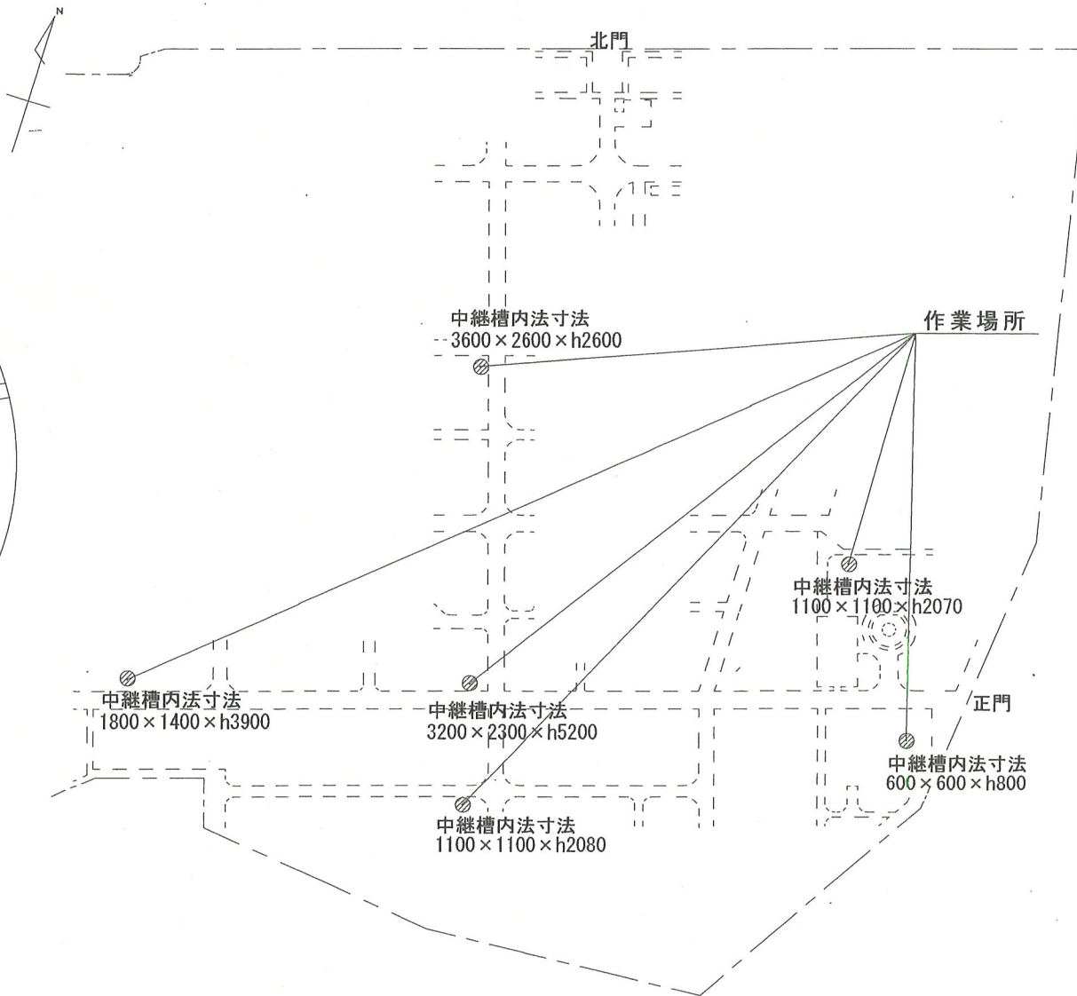
配置図 S=1:4500
