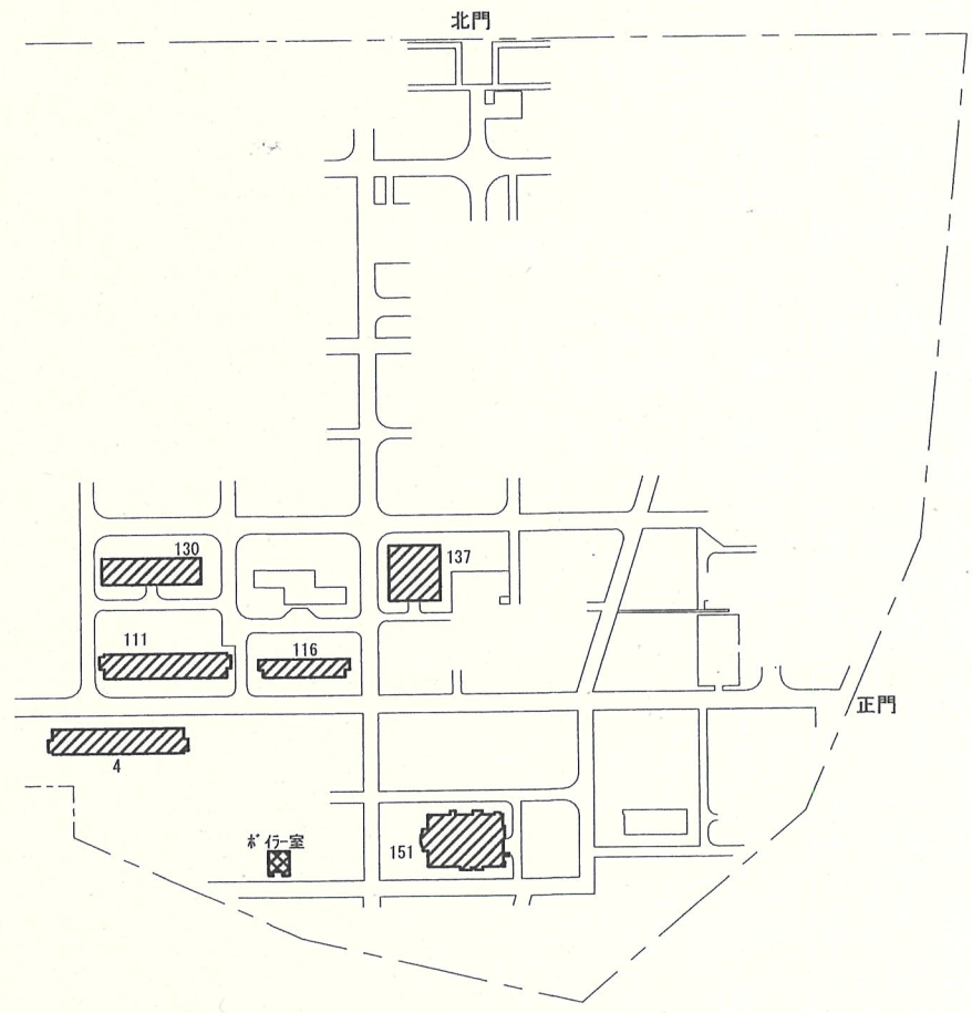
配置図 S=1:5500
