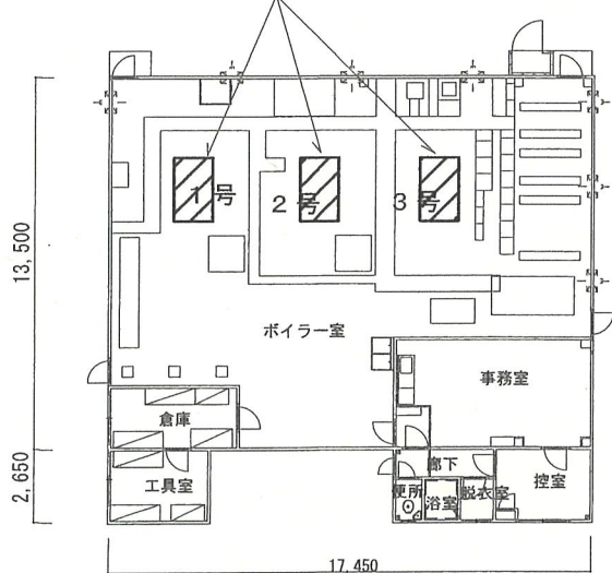
15号建物平面図 S=1/300
