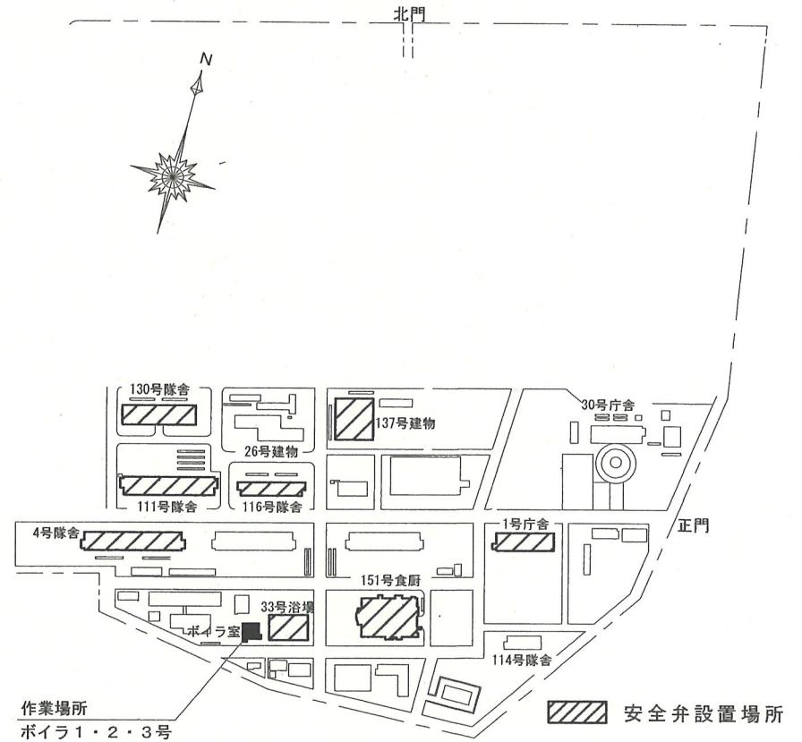
配置図 S=1/6000
