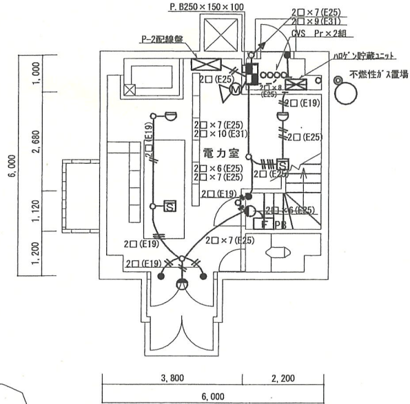
1階平面図
