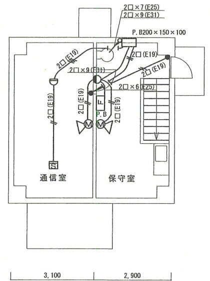
2階平面図
