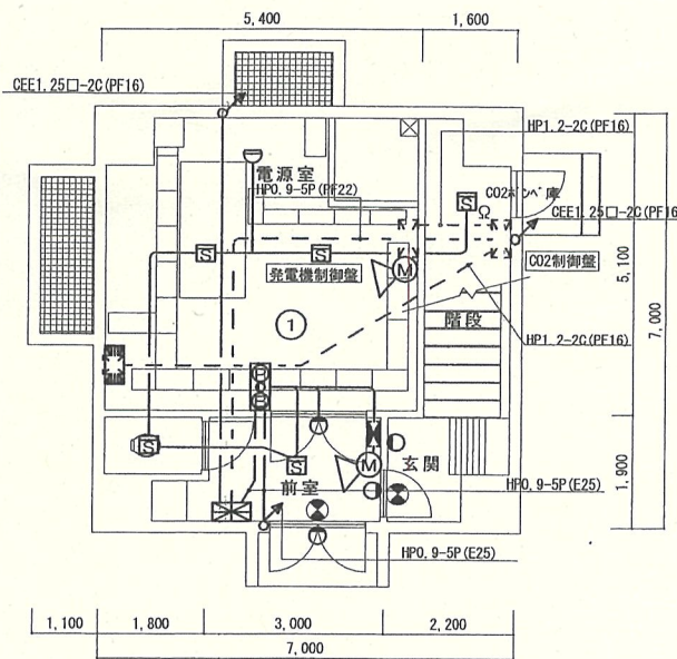
1階平面図
