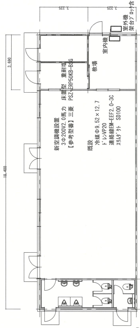
14号建物空調機設置平面図 S=1:150
