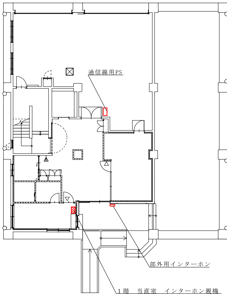
愛媛地方協力本部 1階平面図 S=1/1000
