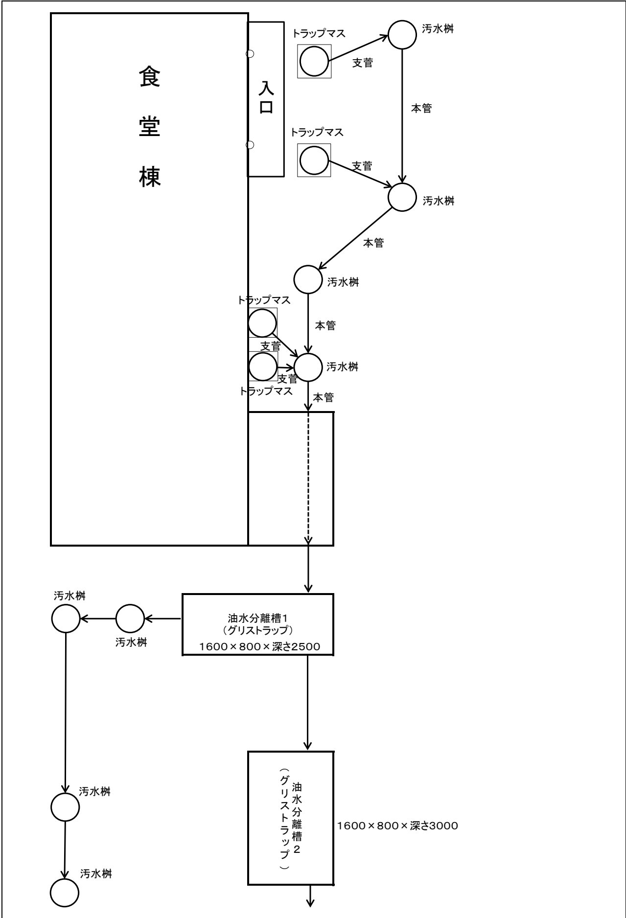
図1ー作業実施場所(油水分離槽)
