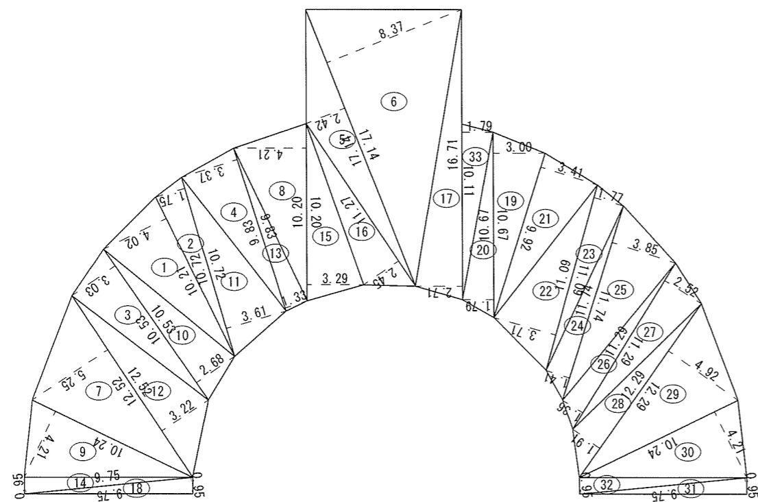
求積図 1/300
