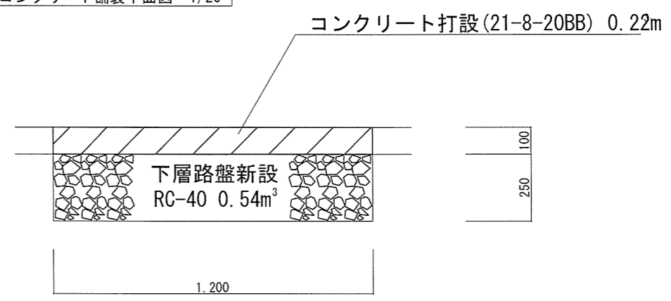
コンクリート舗装断面図 1/20
