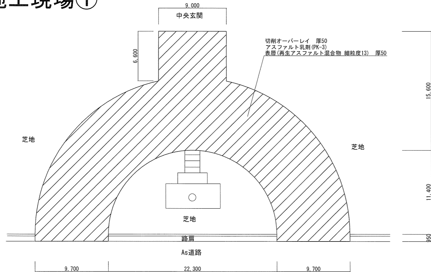
補修配置平面図 1/300
