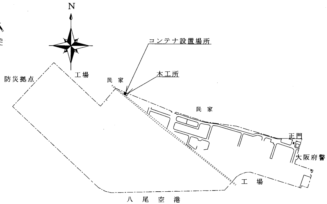
配置図
