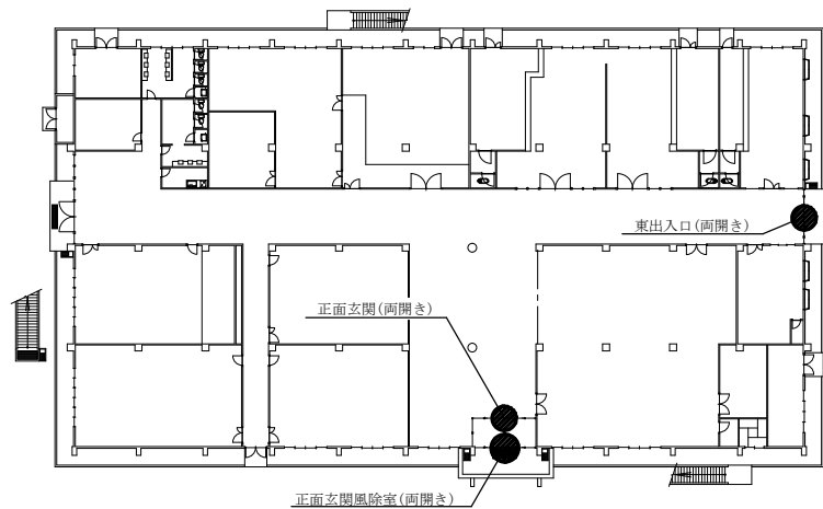
130号建物平面図 S=1/500
