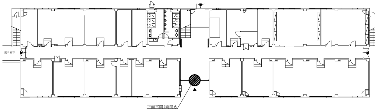
90号建物平面図 S=1/300
