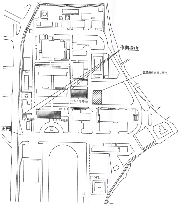
配置図 S=1/3,000
