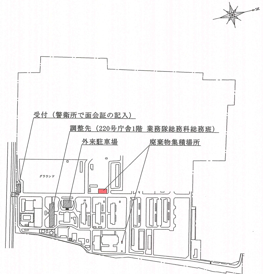
駐屯地配置図 (S=1 : 5000)
