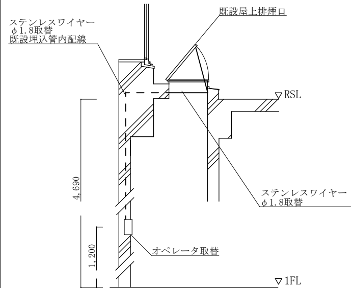
A-A' 断面標準図 S=1/50
