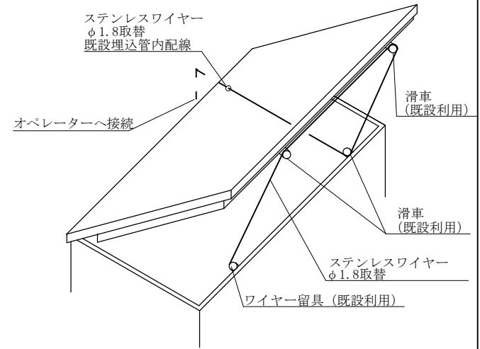
屋上排煙口詳細標準図 S=1/X
