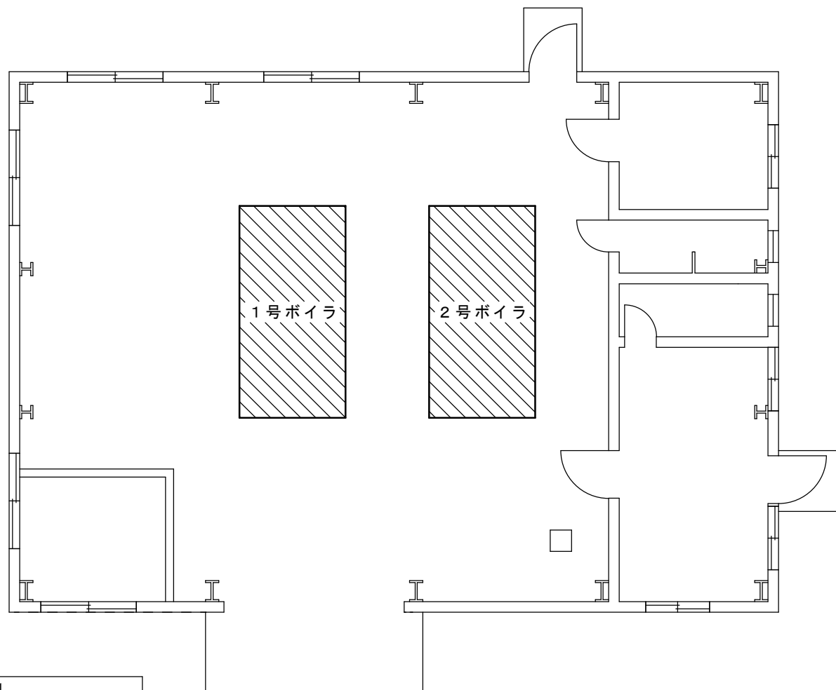
19号建物平面図 S=1/100
