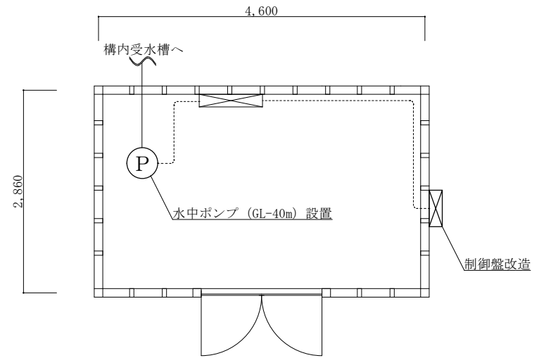
井戸ポンプ室平面図 S = 1 : 75
