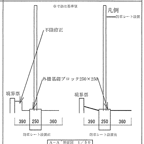
A-A'断面図 1/50
