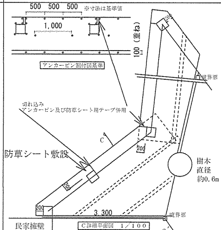
C詳細平面図 1/100
