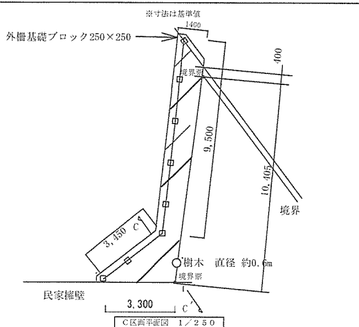
C区画平面図 1/250
