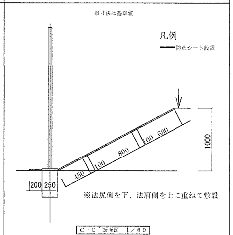
C-C'断面図 1/60
