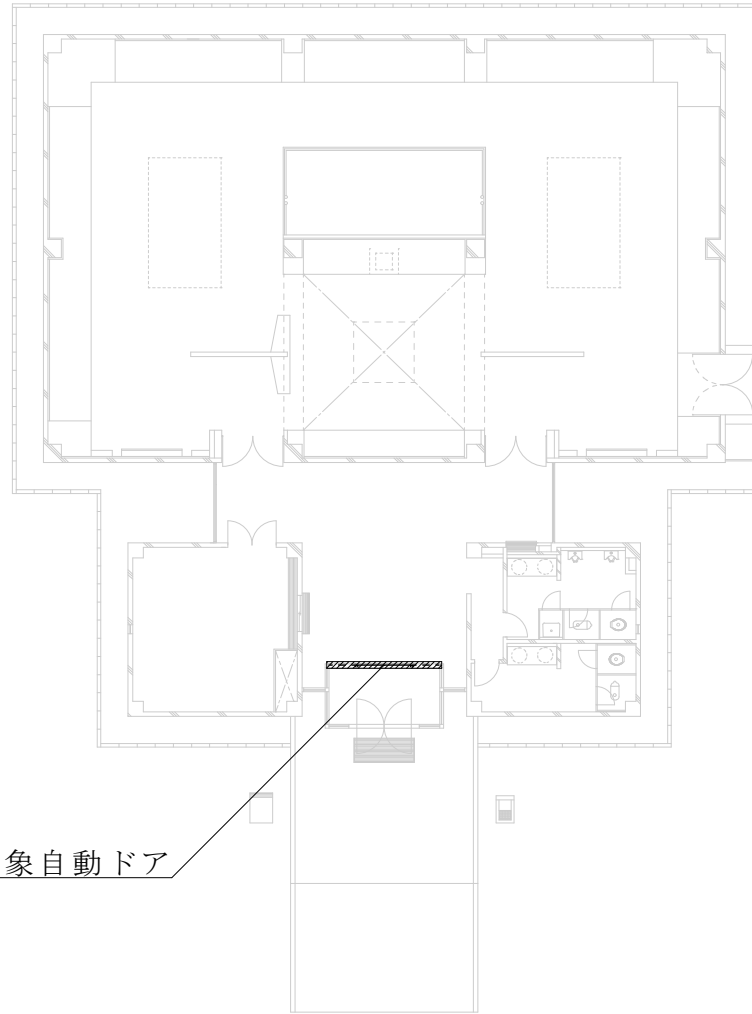
223号建物 平面図 S = 1 / 250
