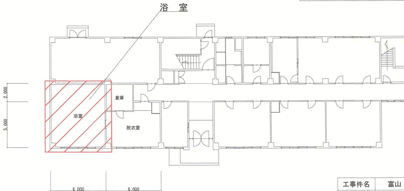
生活隊舎1階配置図 S=1:250
