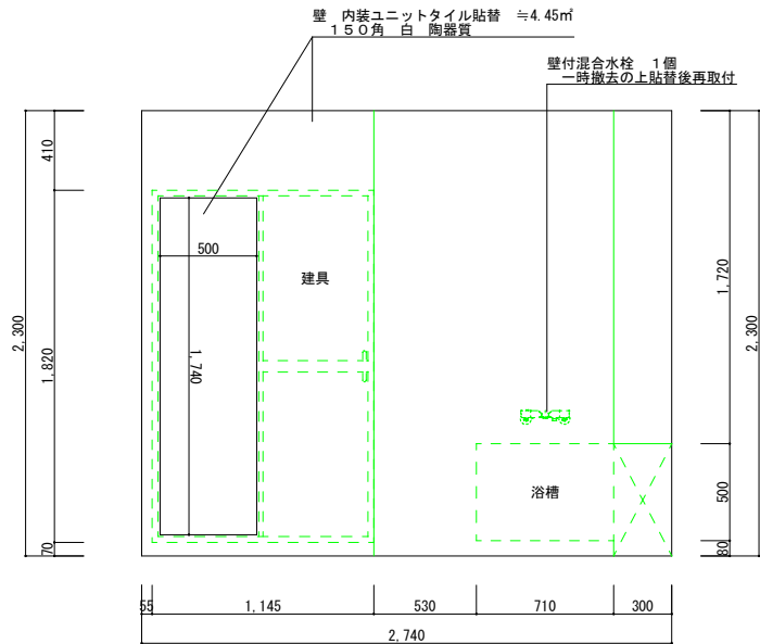
A側展開図(標準) S=1/30
