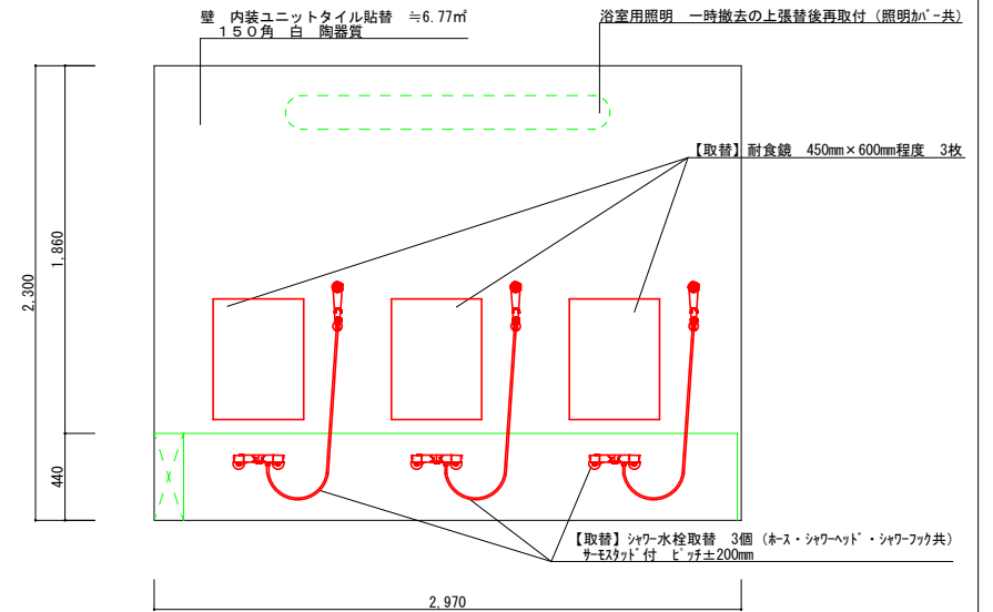
C側展開図(標準) S=1/30
