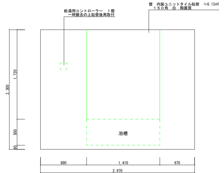
B側展開図(標準) S=1/30
