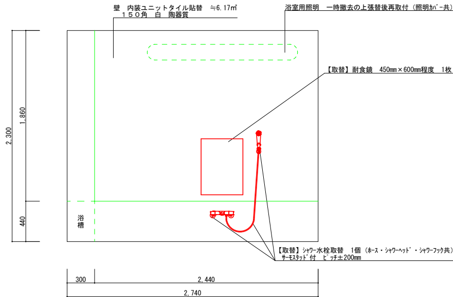
C側展開図(標準) S=1/30
