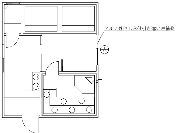
189号建物平面図 S=1/100
