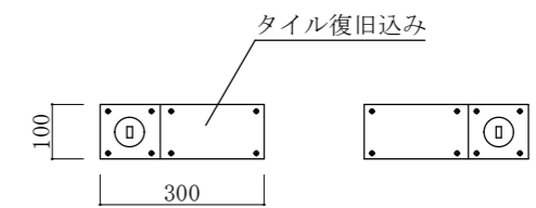
フロアヒンジ平面図 S=1/15
