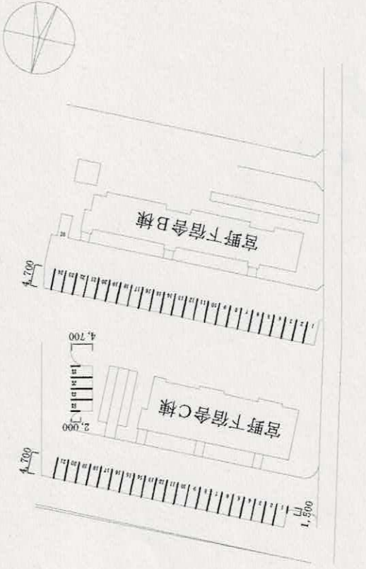
宮野下宿舎B・C棟配置図 S=1/800
