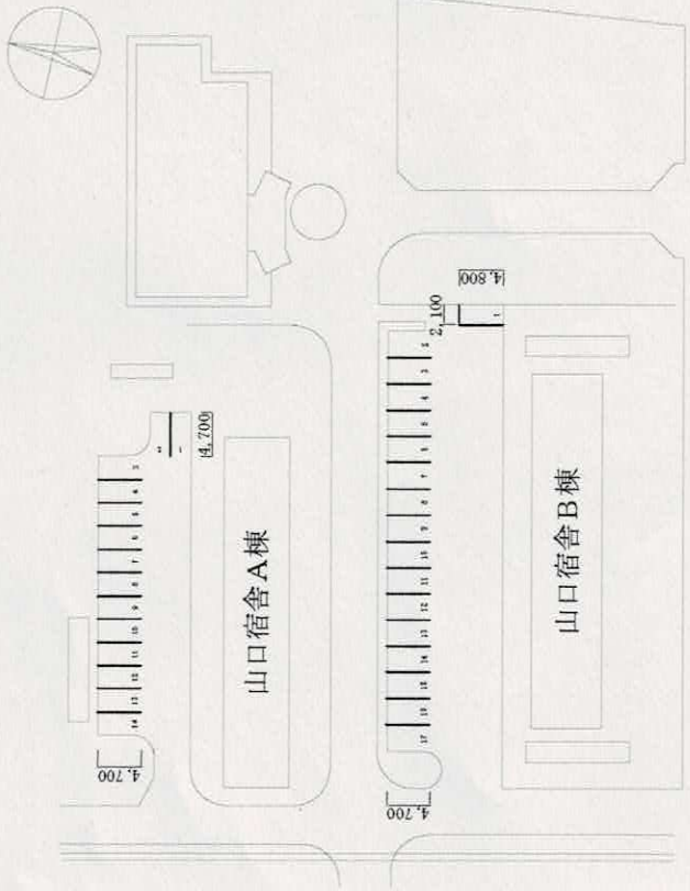
山口宿舎A・B棟配置図 S=1/600
