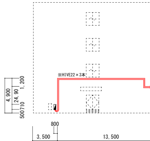
室外機電源線西立面図 S=300
