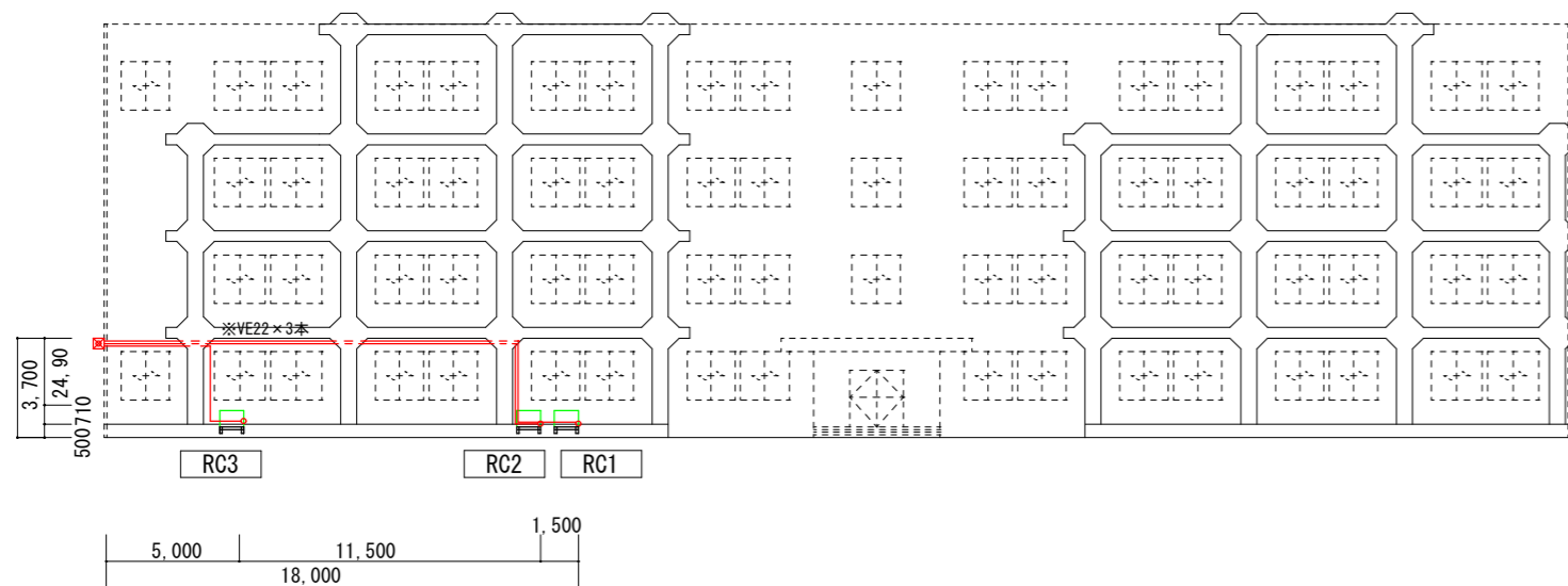
室外機電源線北立面図 S=300
