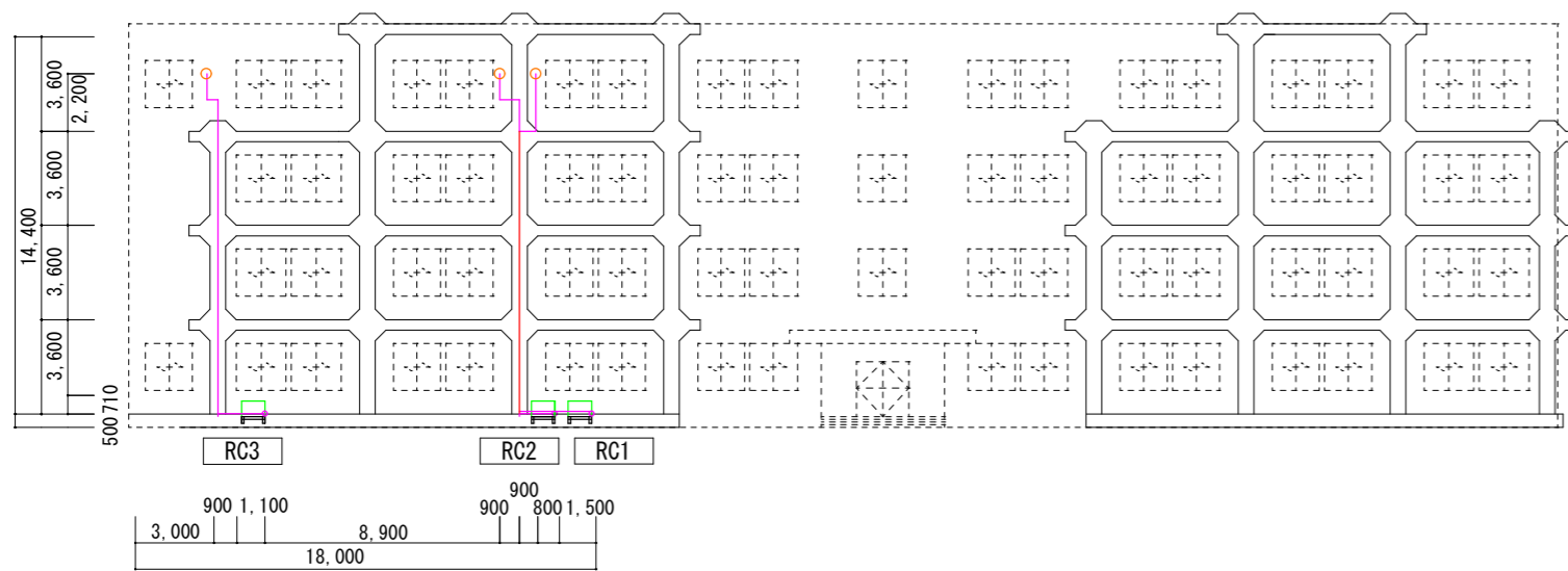
空調付帯配管類北立面図 S=300
