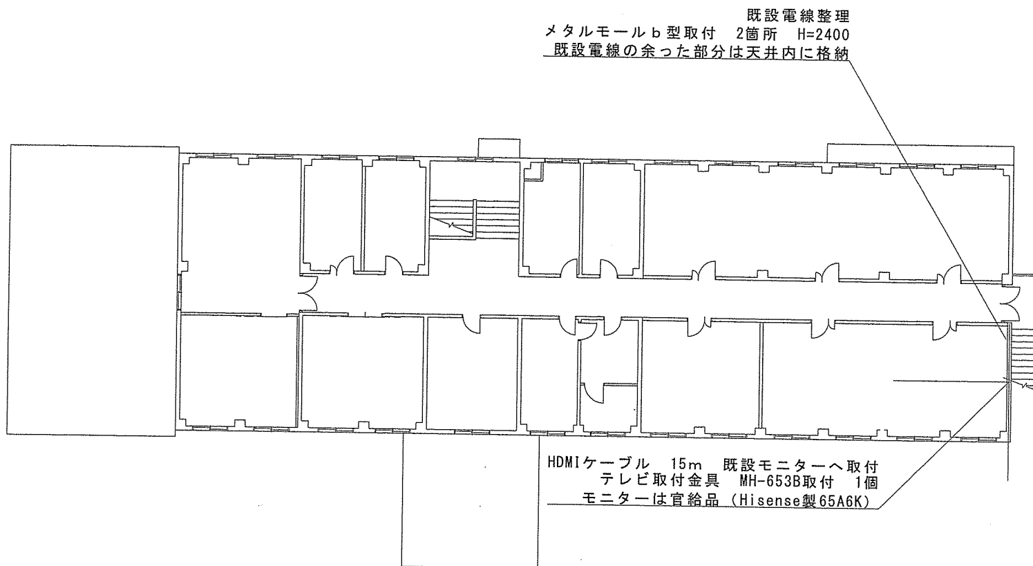
1号本部隊舎2階詳細図 (1/200)
