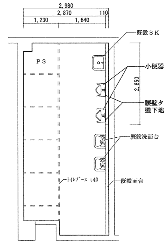
1階便所平面図 S = 1 / 80
