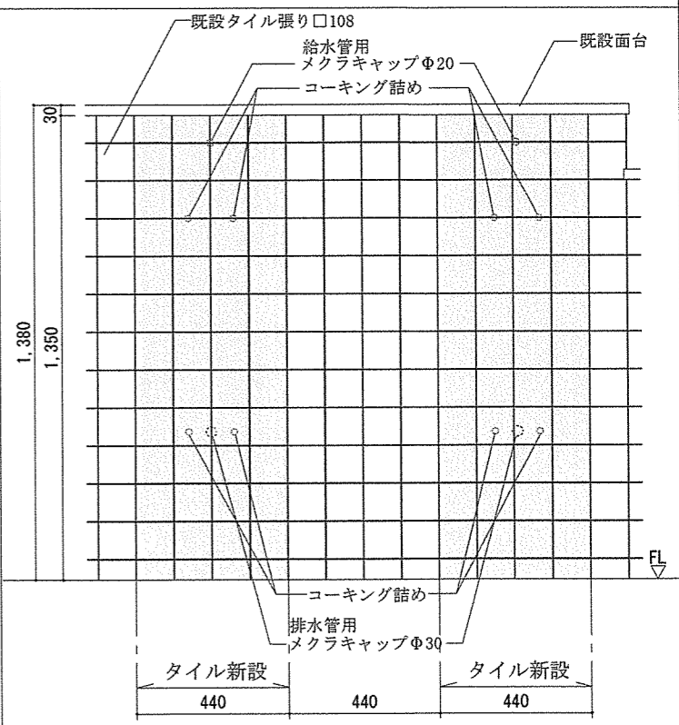
東面小便器改修後展開図 S = 1 / 20
