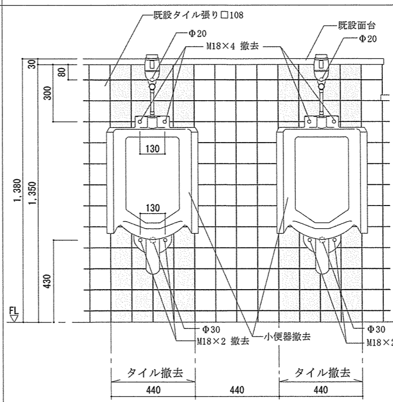
東面小便器改修前展開図 S = 1 / 20
