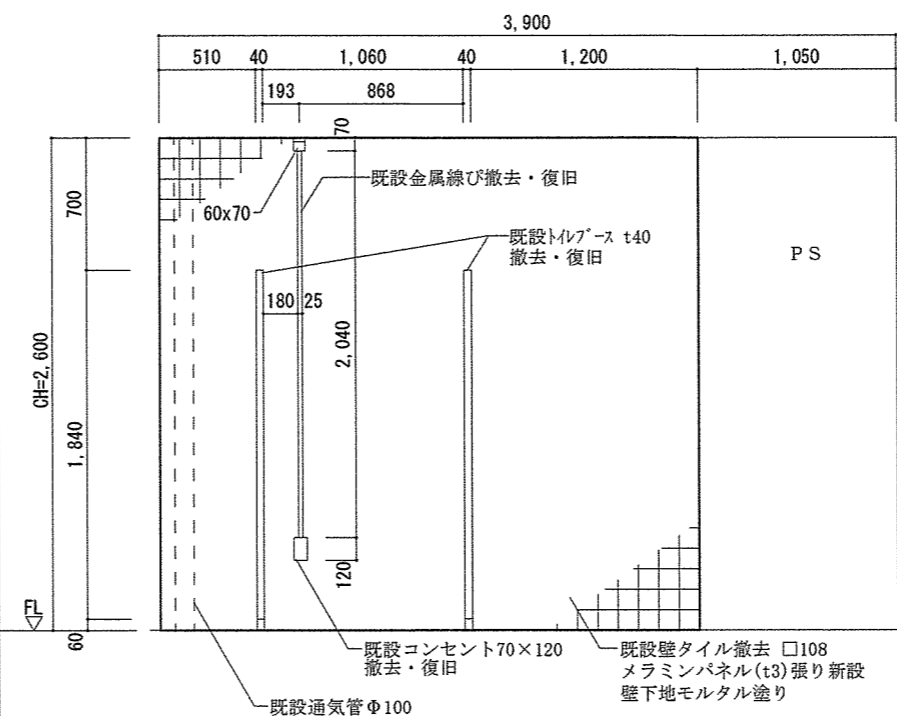
便所B面改修展開図 S = 1 / 40
