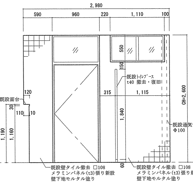
便所D面改修展開図 S = 1 / 40
