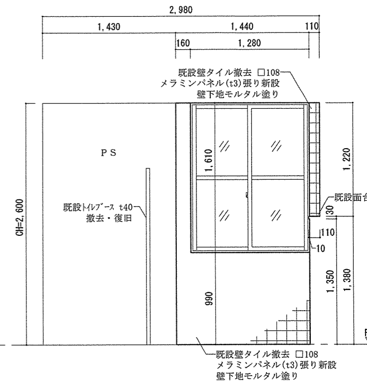
便所C面改修展開図 S = 1 / 40
