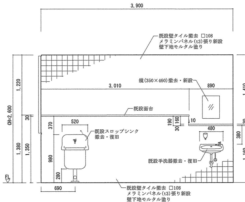
便所A面改修展開図 S = 1 / 40
