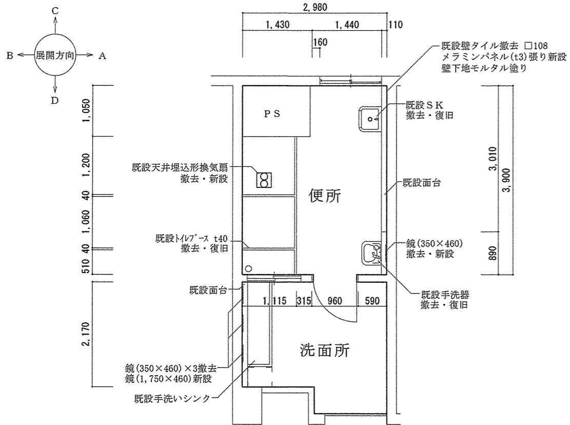
3階便所・洗面所①平面図 S = 1 / 80
