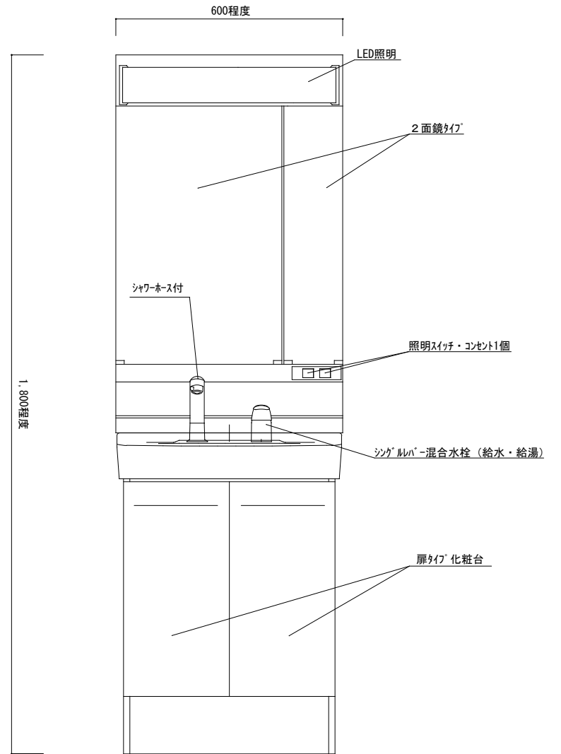
洗面化粧台姿図 (標準) S=1/X
