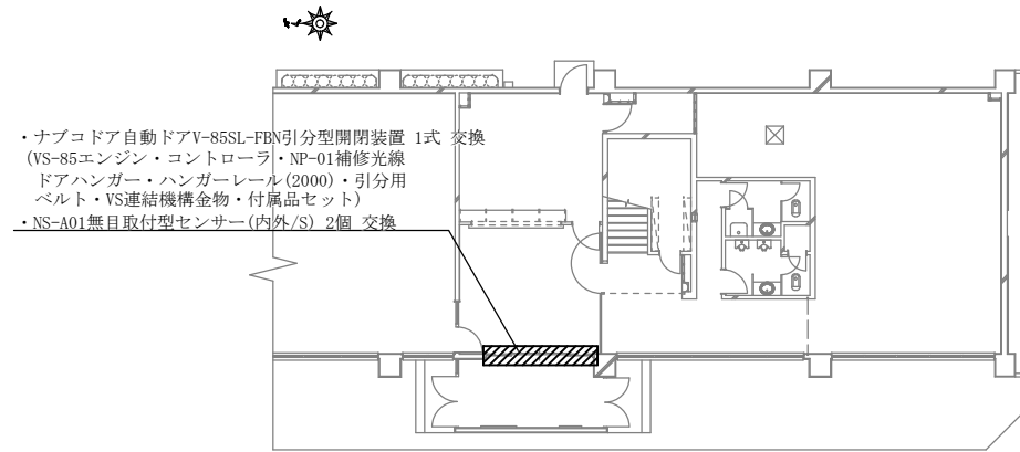
139号建物1階平面図 S=1/200
