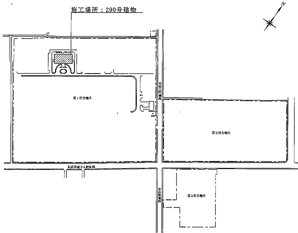
配置図 S=NS
