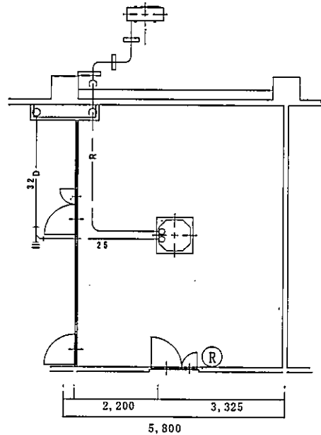
290号建物空調機配置図 (S=1/100)
