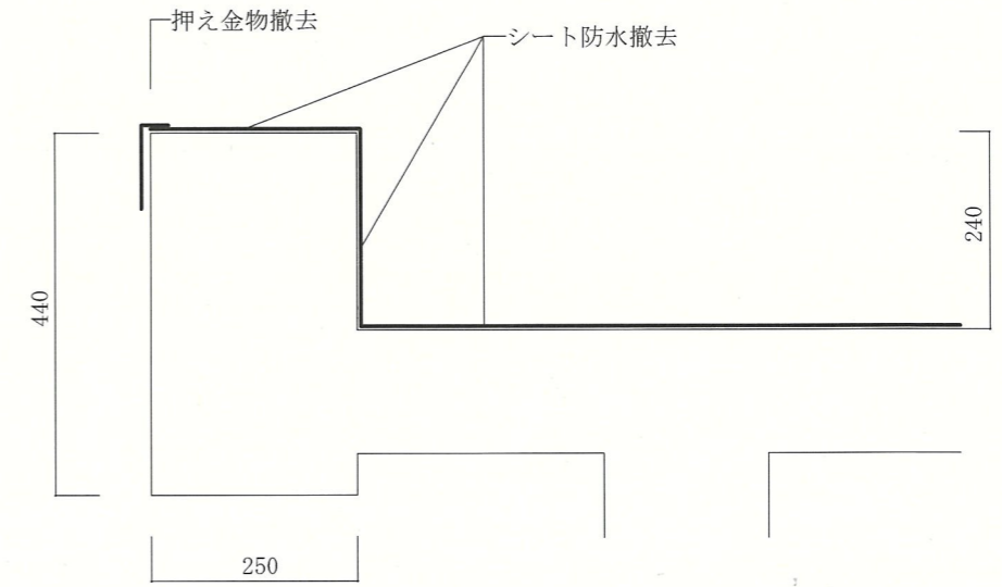
改修前A-A'断面図 S=1/10
