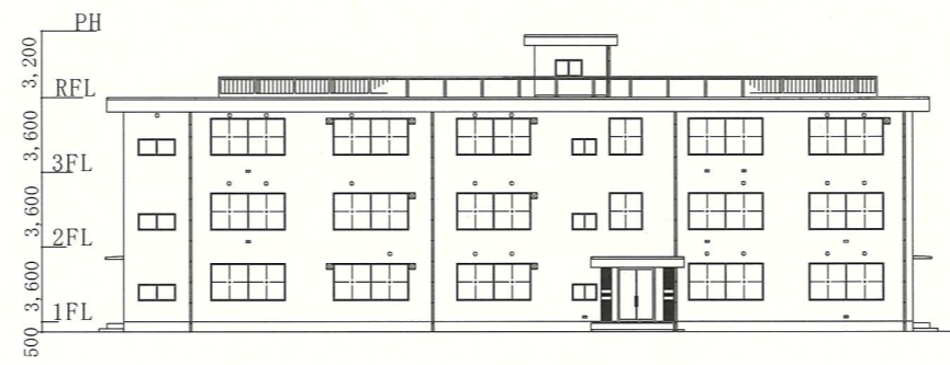
北側立面図 S=1/400
