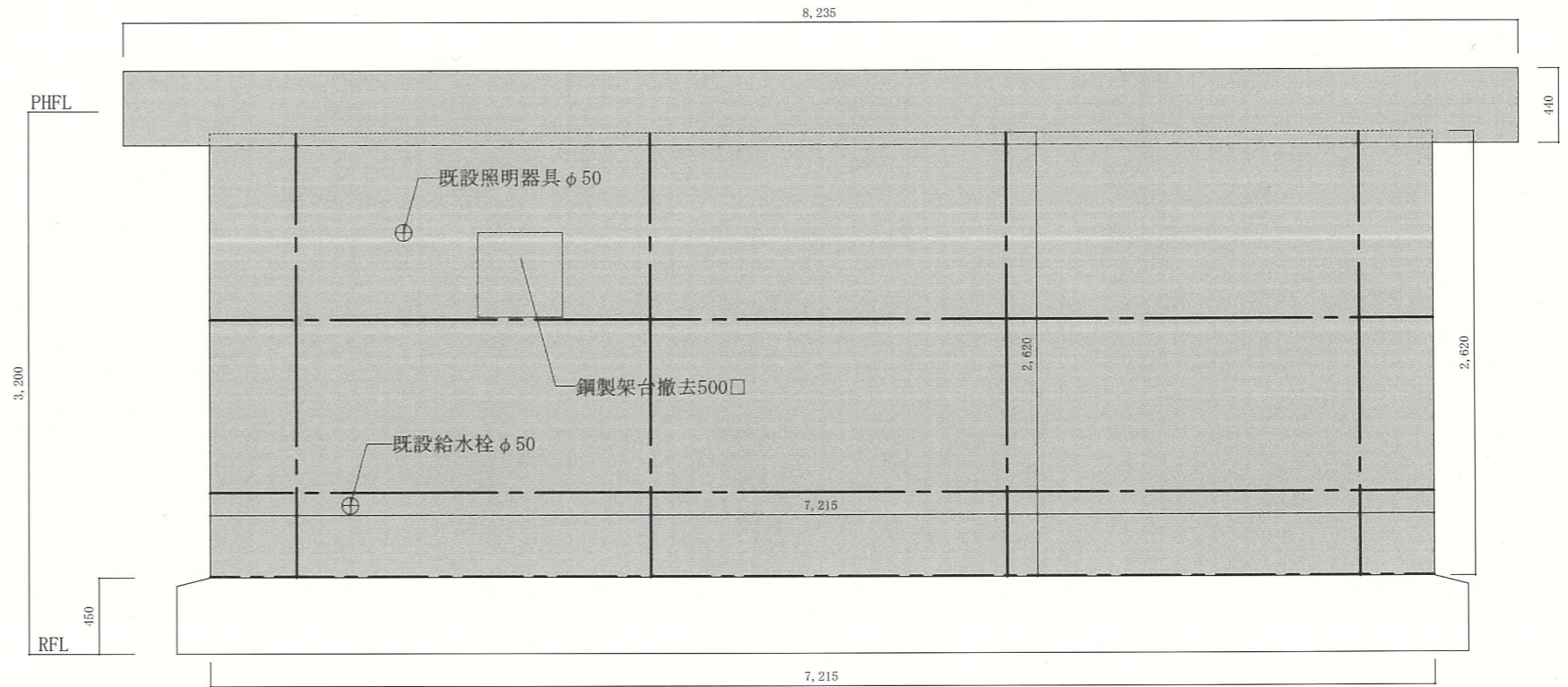
東面立面図
