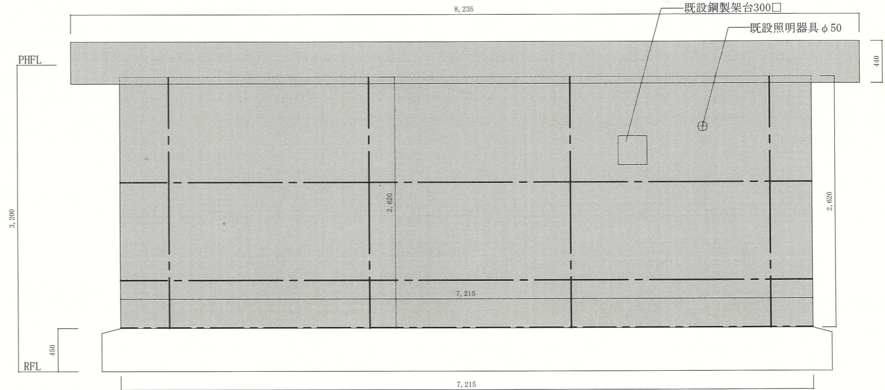
西面立面図
