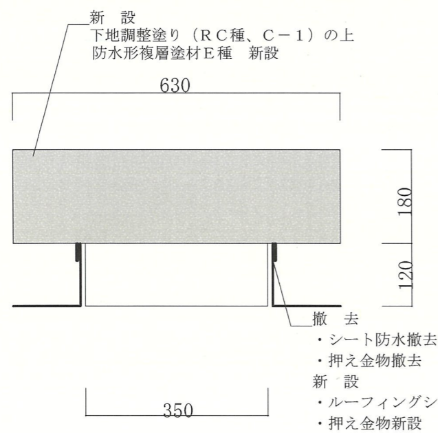
機械基礎①断面図 S=1/10
