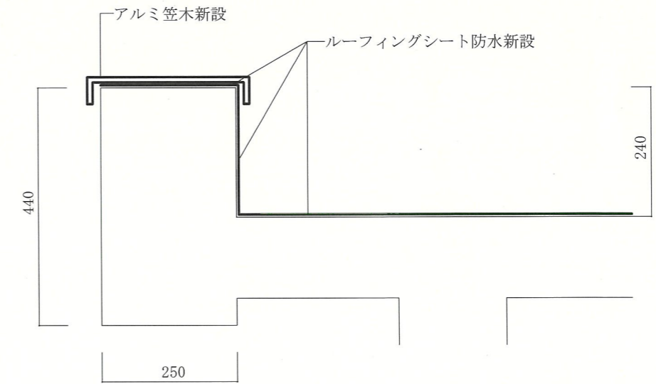
改修後A-A'断面図 S=1/10
