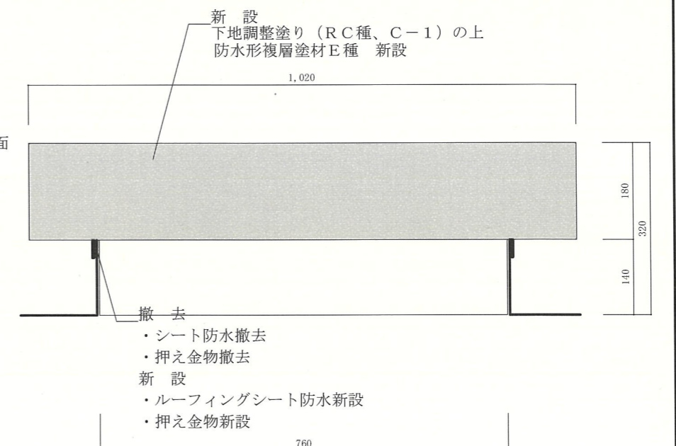
機械基礎④断面図 S=1/10
