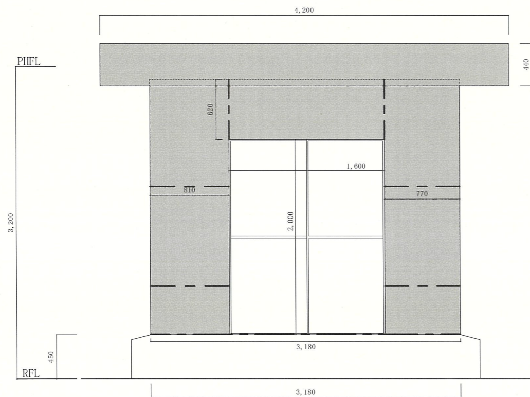
南面立面図
