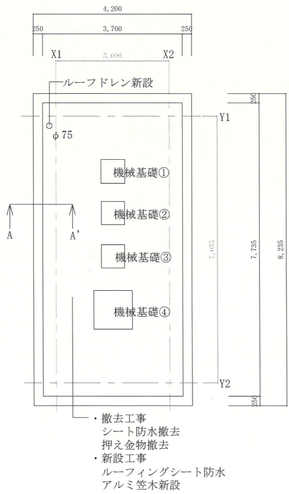
PH屋根伏図 S=1/100
