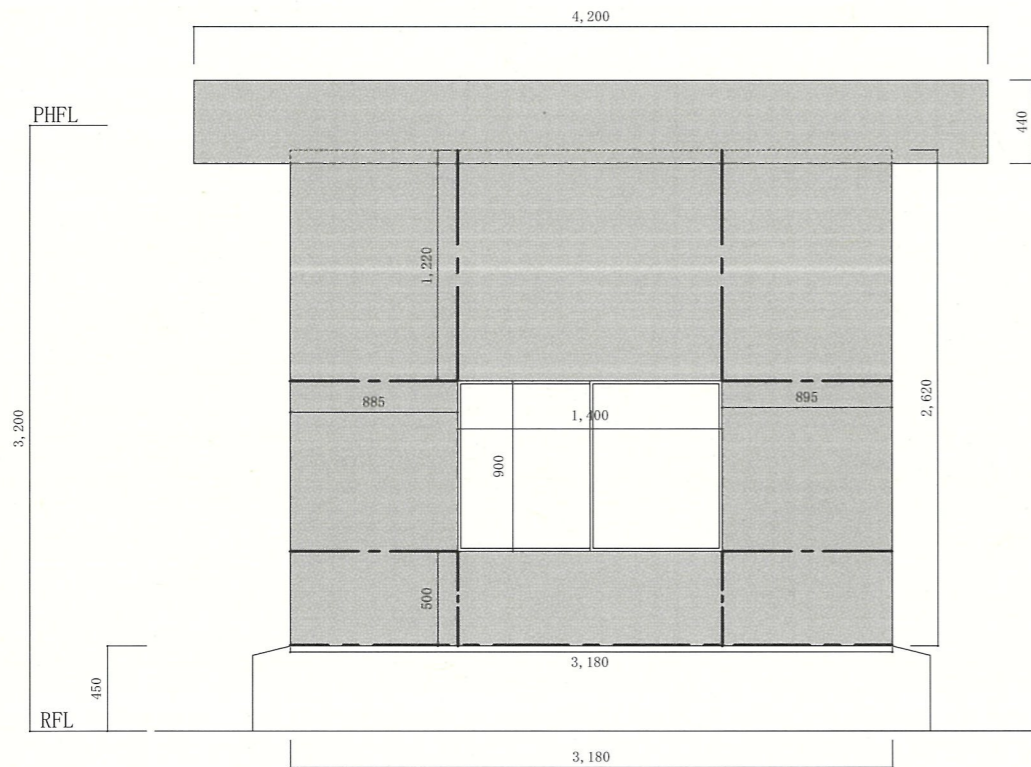
北面立面図
