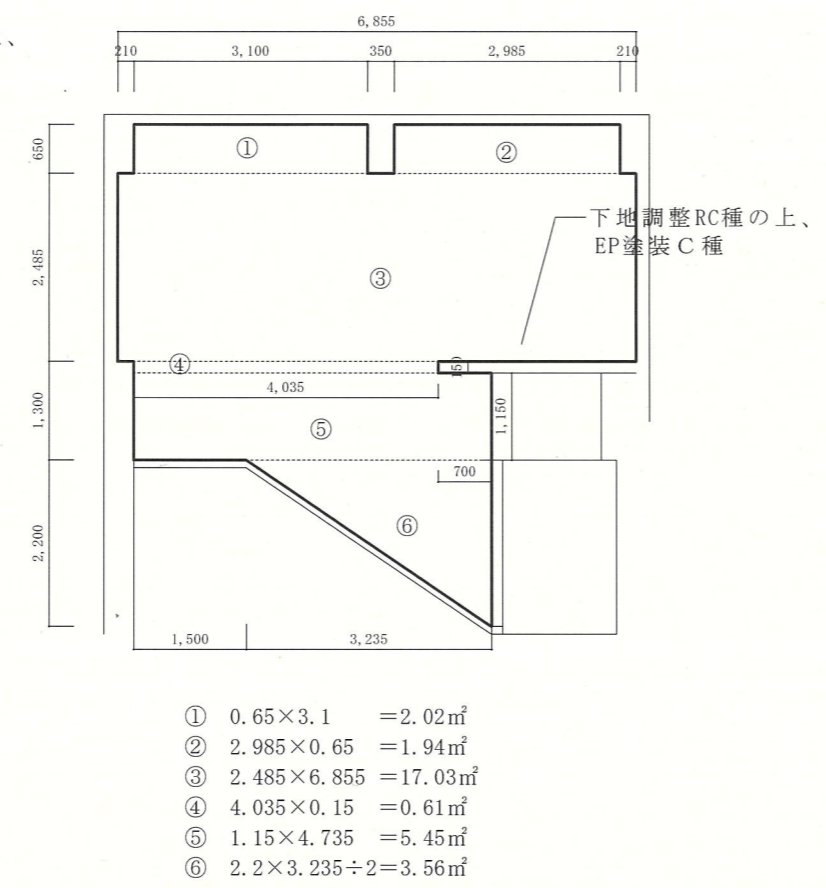
B面展開図 S=1/100
