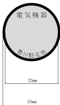
製作図
