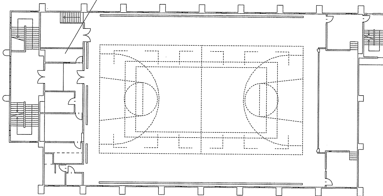
24号体育館2階平面図
