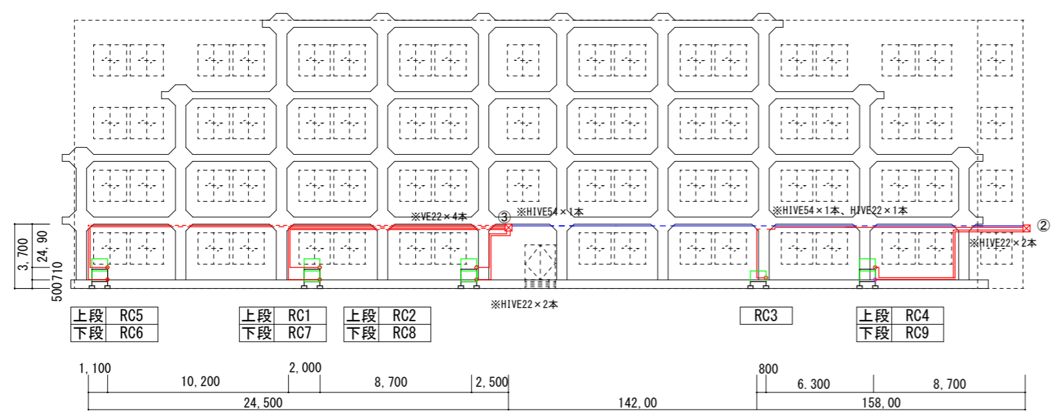
室外機電源線南立面図 S=300
