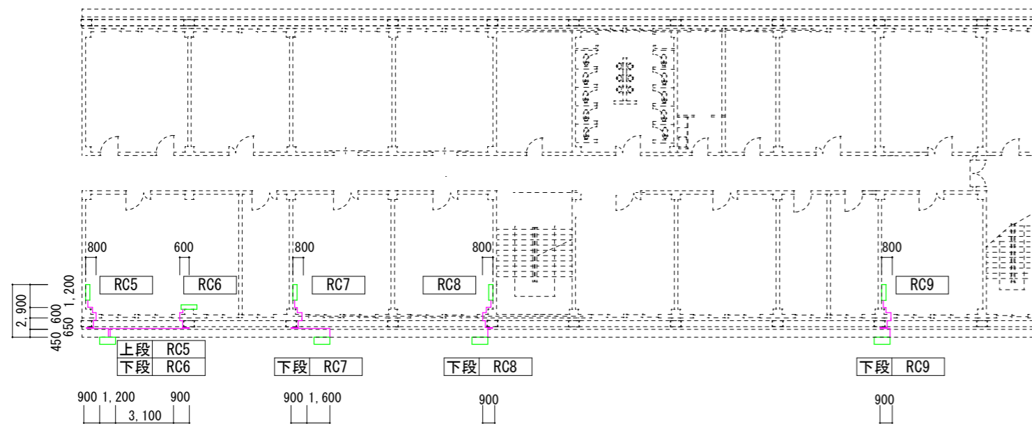
4 F 空調付帯配管類平面図 S=300
