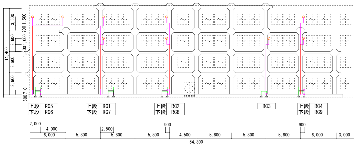
空調付帯配管類南立面図 S=300
