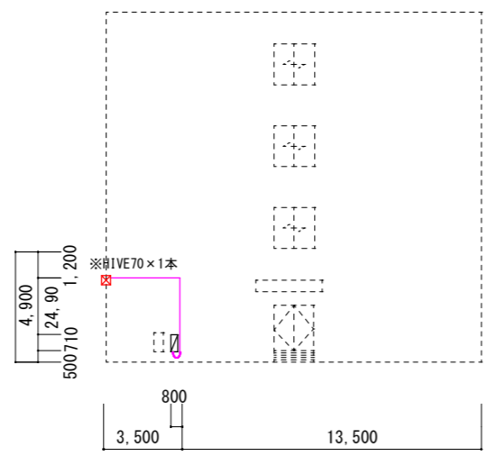
室外機電源線西立面図 S=300
