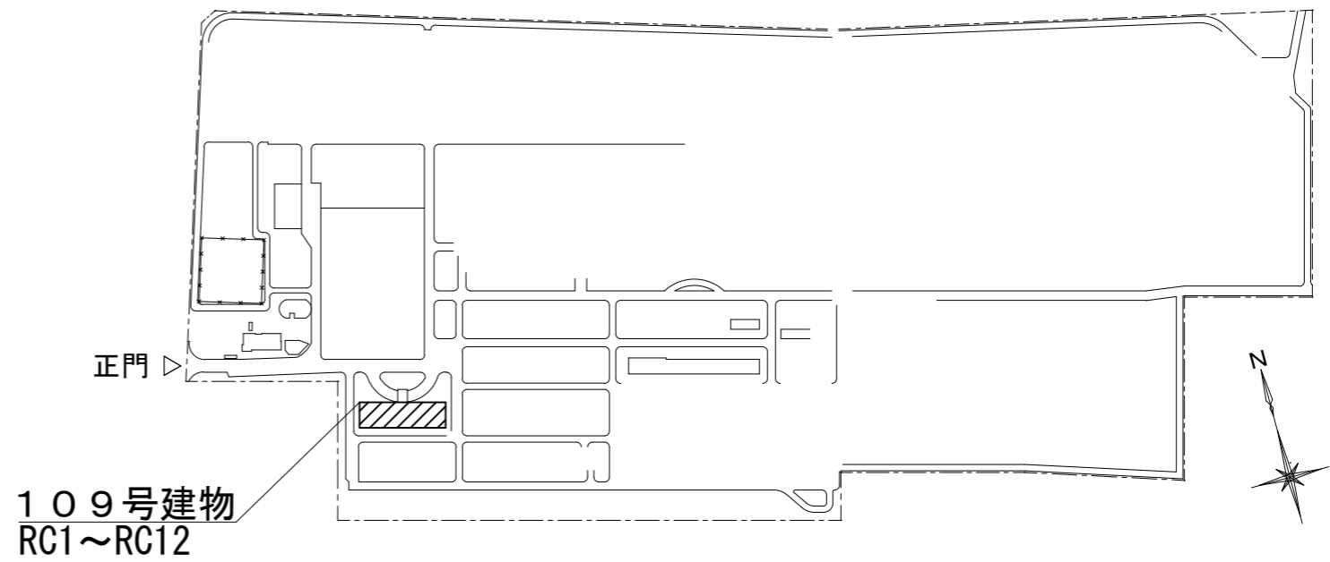
米子駐屯地 配置図 1:6000
